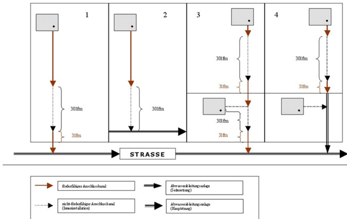
Abbildung 1 (Haus)Anschlusskanäle - Fallbeispiele
