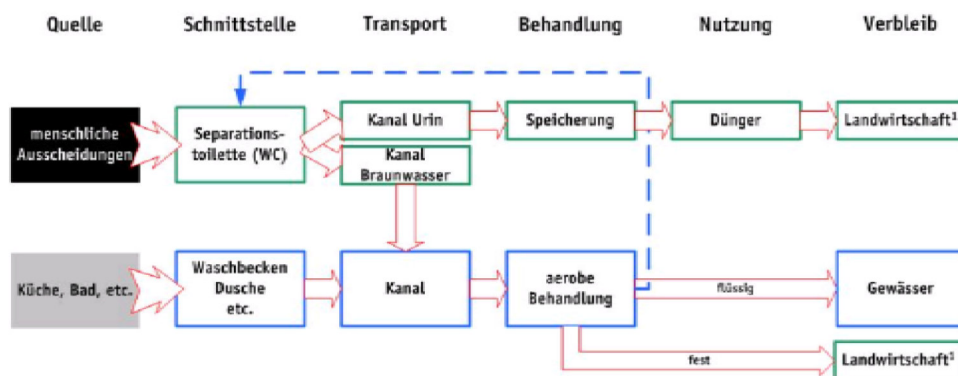
Abbildung 3 Variante B für Beispiel kreislaforientierte Abwassersysteme für Einzelanlagen
