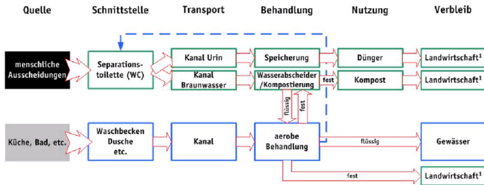
Abbildung 2 Variante A für Beispiel kreislaforientierte Abwassersysteme für Einzelanlagen
